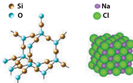
Мал. 60. Склад: кварцу — речовини атомної будови (а) та кухонної солі — речовини йонної будови (б)
