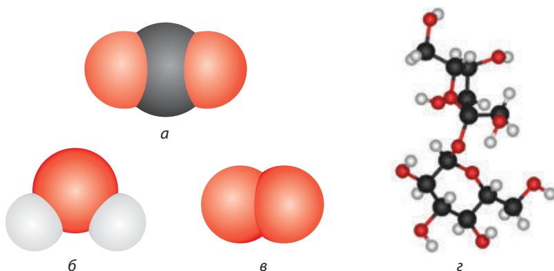
Мал. 51. Моделі молекул: а — вуглекислого газу; б — води; в — кисню; г — сахарози.
