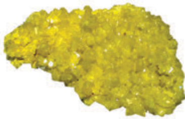
Мал. 37. Рідкісні приклади чистих речовин у природі: а — самородне золото; б — самородна сірка
