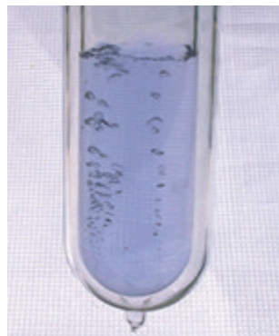
Мал. 80. Рідкий кисень має блакитне забарвлення
