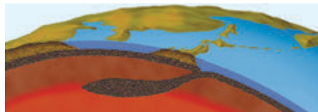
Літосфера — 49 %
