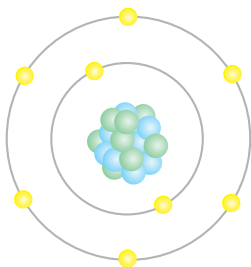
Мал. 84. Модель атома Оксигену
