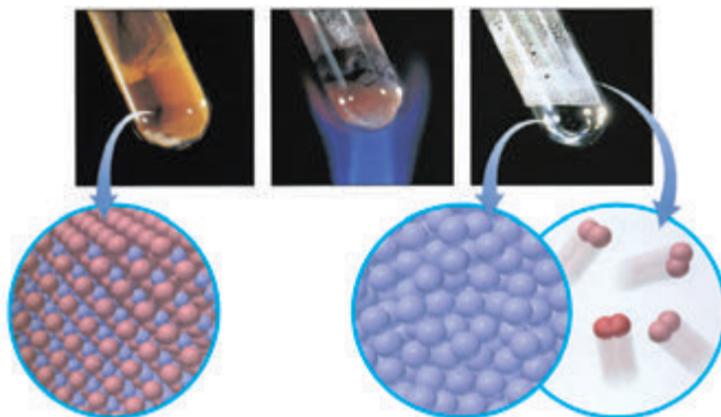
Мал. 90. При прожарюванні червоного ртуті(II) оксиду утворюється рідка сріблеста ртуть і газуватий кисень
