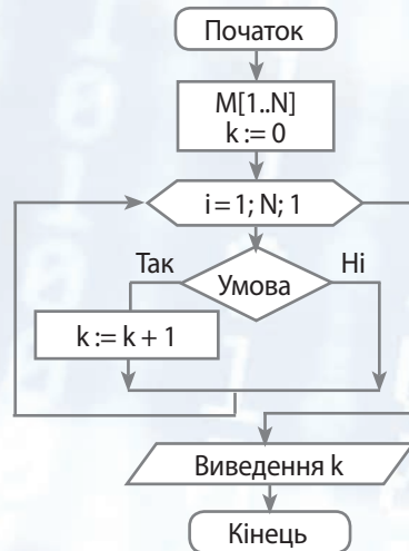
Знаходження кількості елементів одновимірного масиву M[1..N] , що задовольняють певній умові
