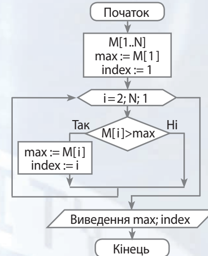
Знаходження значення і першого індексу найбільшого елемента в одновимірному числовому масиві M[1..N]
