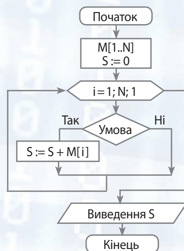
Знаходження суми S елементів одновимірного числового масиву M[1..N] , що задовольняють певній умові
