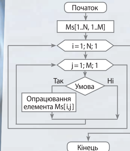
Опрацювання елементів двовимірного масиву Ms[1..N, 1..M] , які задовольняють певній умові
