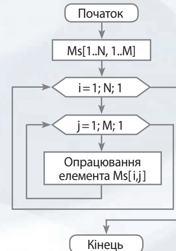
Опрацювання елементів двовимірного масиву Ms[1..N, 1..M]
