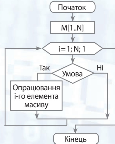
Опрацювання елементів одновимірного масиву M[1..N] , які задовольняють певній умові
