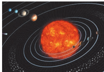
Рис. 27.4 Комп'ютерна модель Сонячної системи
