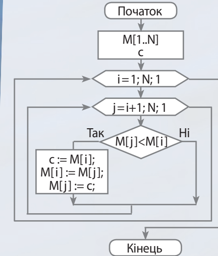
Упорядкування за зростанням (неспаданням) елементів одновимірного масиву M[1..N]
