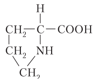
Пролін (Про)
