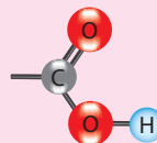
Карбоксильна
