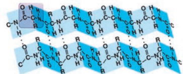
\beta -складчаста структура
