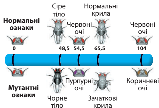
Мал. 31.4. Карта однієї з хромосом дрозофіли
