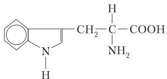
Триптофан (Трп)
