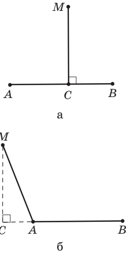
Рис. 205. Визначення відстані від точки до відрізка
