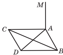
ABDC — ромб
