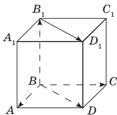
Рис. 265. Компланарні і некопланарні вектори
