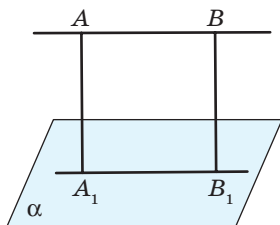
Рис. 152. До обґрунтування визначення відстані від прямої до паралельної їй площини
