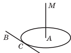
BC — дотична до кола з центром A
