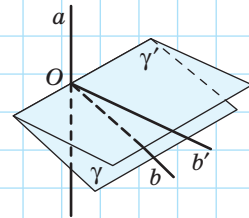
Рис. 135. До доведення єдиності перпендикулярної площини
