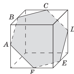
Рис. 103. Переріз куба
