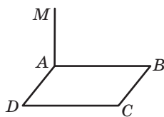
ABCD — прямокутник
