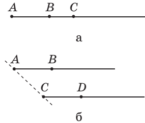
Рис. 242. Співнапрямлені промені
