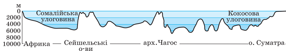
Рис. 1. Профіль океанічної улоговини Індійського океану (у районі 5° пд. ш.).
