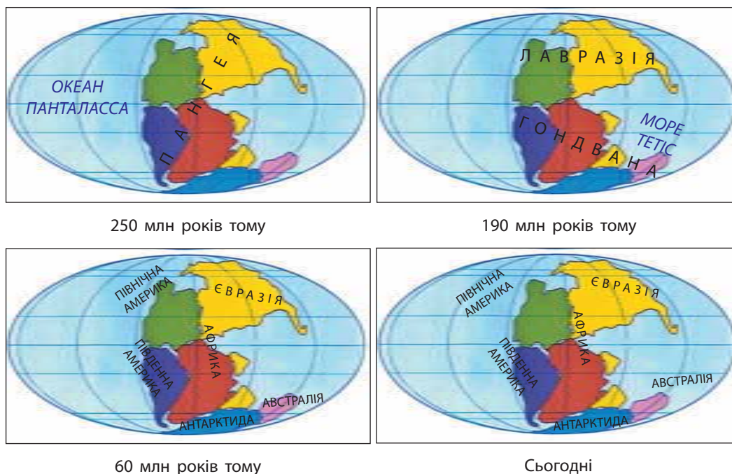
Рис. 2. Дрейф континентів.
