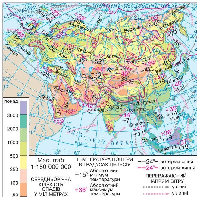
Рис. 1. Клімат Євразії.
