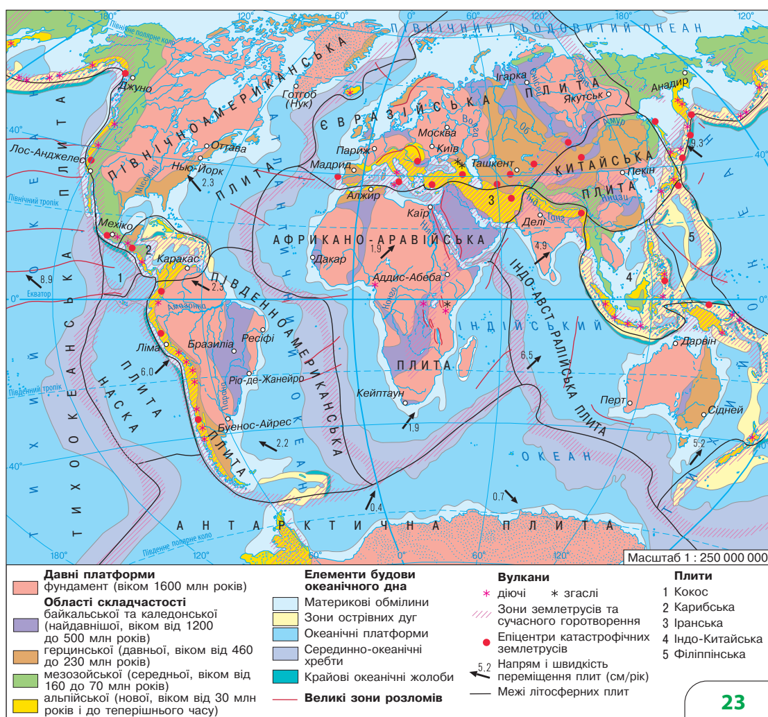
Рис. 1. Будова земної кори.
