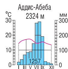
Рис. 1. Кліматичні діаграми.
