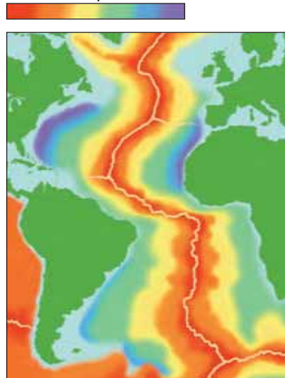
Рис. 3. З усіх серединно-океанічних хребтів найкраще вивчений Серединно-Атлантичний хребет, який є стержневим елементом рельєфу дна Атлантичного океану. Велетенська структура з відносною висотою до 4 км простягається від острова Ісландія на півночі до 65° пд. ш. Найбільшої ширини хребет сягає в Південній Атлантиці — до 1500 км.
