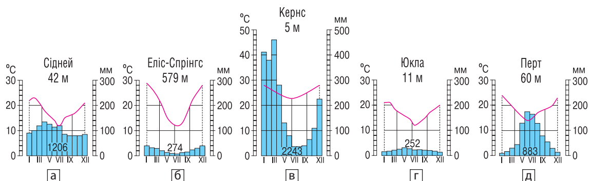
Рис. 2. Кліматичні діаграми.
