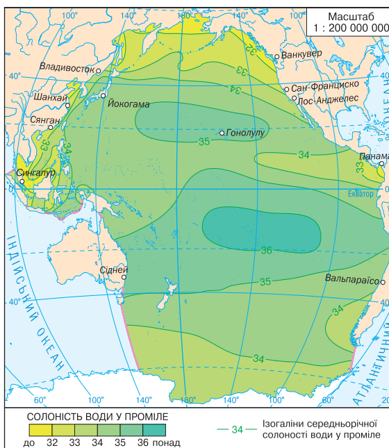
Рис. 4. Солоність поверхневих вод.
