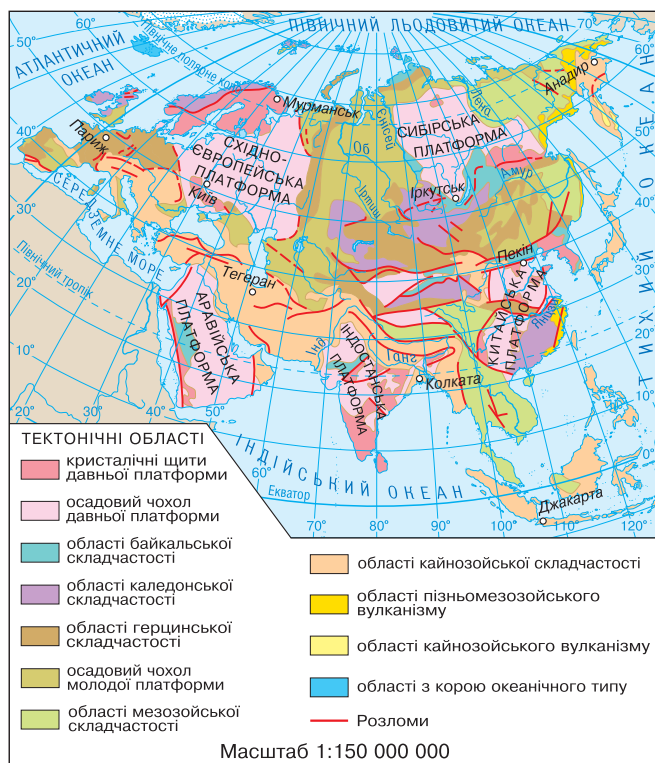
Рис. 1. Будова земної кори Євразії.
