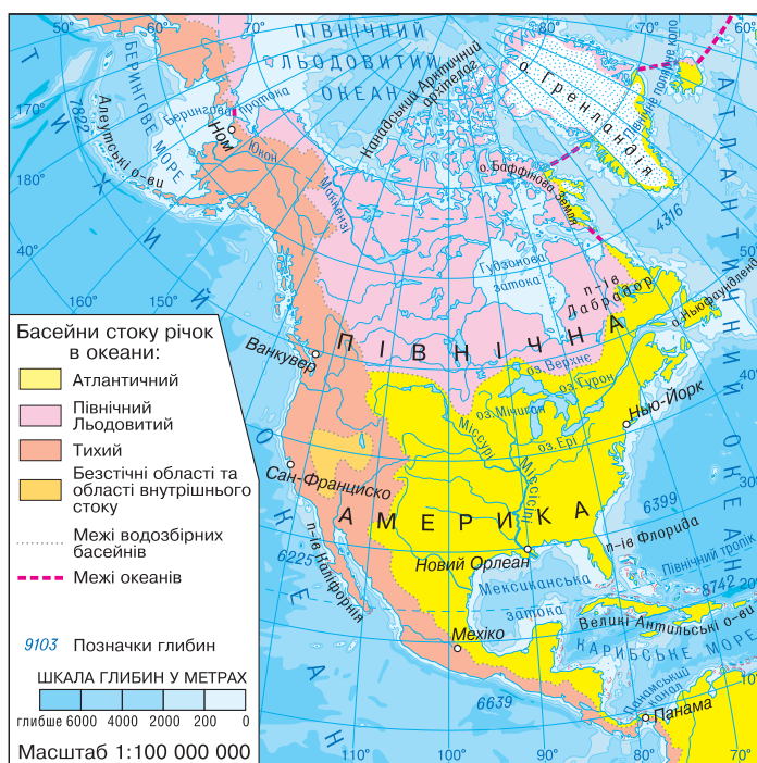
Рис. 1. Басейни стоку річок в океани.
