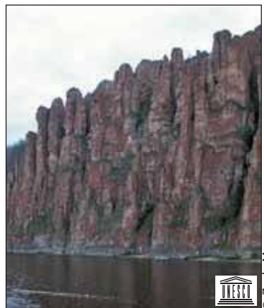
Рис. 3. «Ленські стовпи» — геологічне утворення та однойменний природний парк на березі річки Лени. Тут поширені численні останці від руйнування корінних порід, що утворюють «колонади», «вежі», «арки», «собори» та інші химерні фігури.
