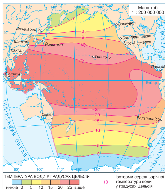
Рис. 3. Температура поверхневих вод.
