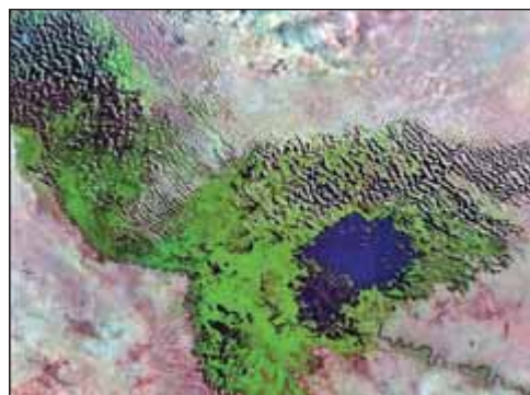
Рис. 5. Озеро Чад.
