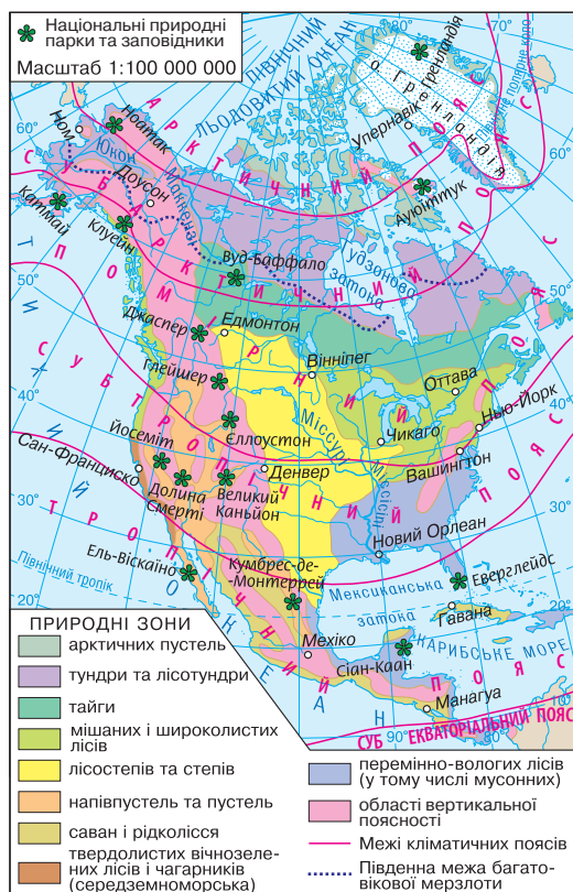
Рис. 1. Природні зони Північної Америки.
