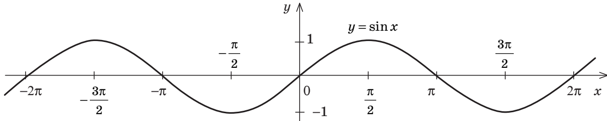
Властивості функції y = \sin x
