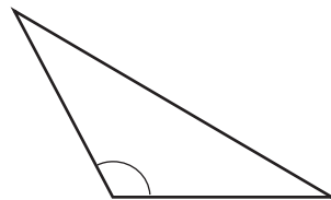
Тупокутний
