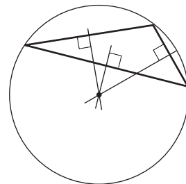
Поза трикутником
