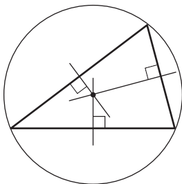
Усередині трикутника
