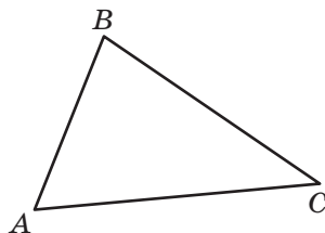
Рис. 54. Трикутник ABC
