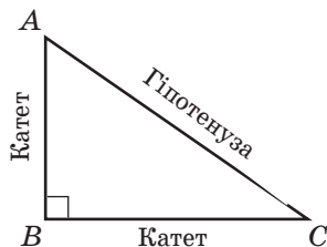
Рис. 147. Прямокутний трикутник
