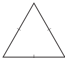
Рис. 82. Рівносторонній трикутник
