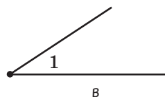
Рис. 17. Позначення кута
